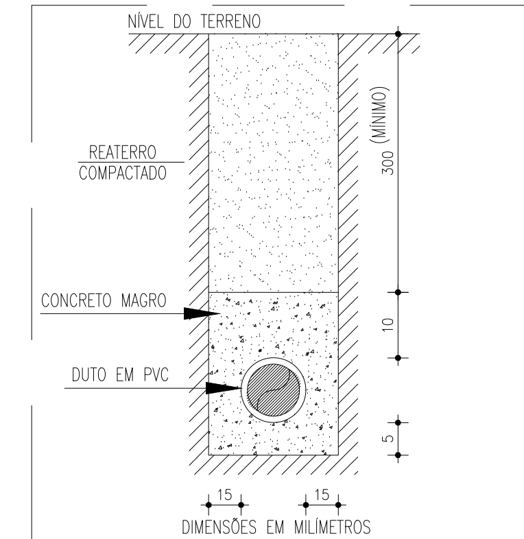
DETALHE ENVELOPAMENTO ESCALA S/E
