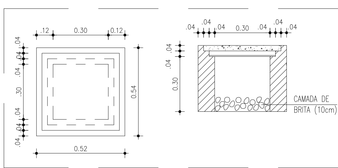
DETALHE CAIXA DE ALVENARIA 30X30X30 CM ESCALA S/E
