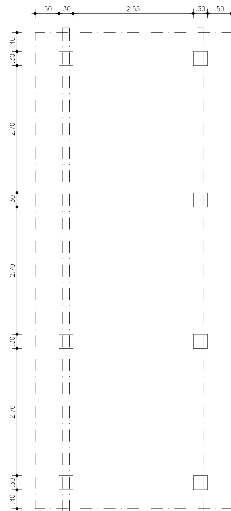
PERGOLADO PLANTA BAIXA NIVEL PILARES
