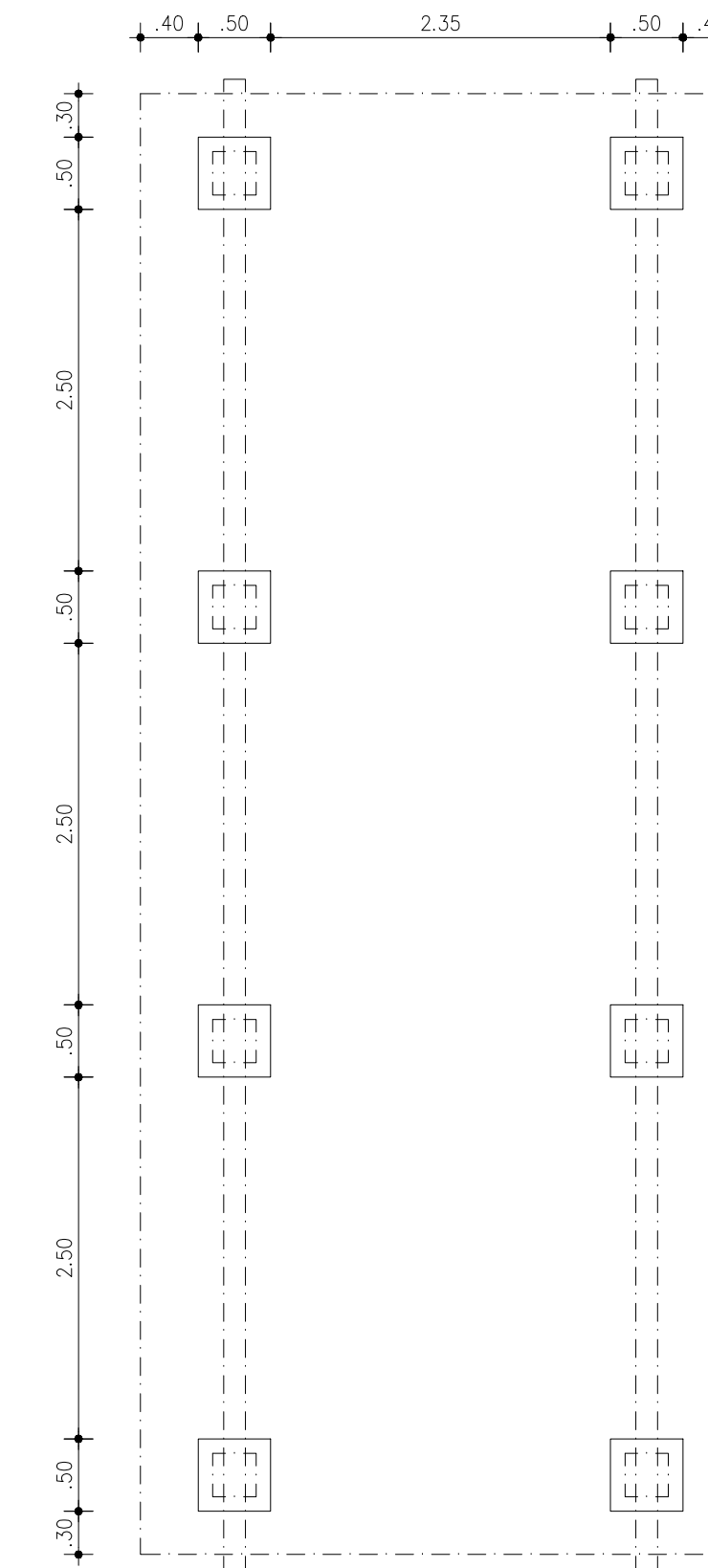
PERGOLADO PLANTA BAIXA NIVEL FUNDAÇÃO
