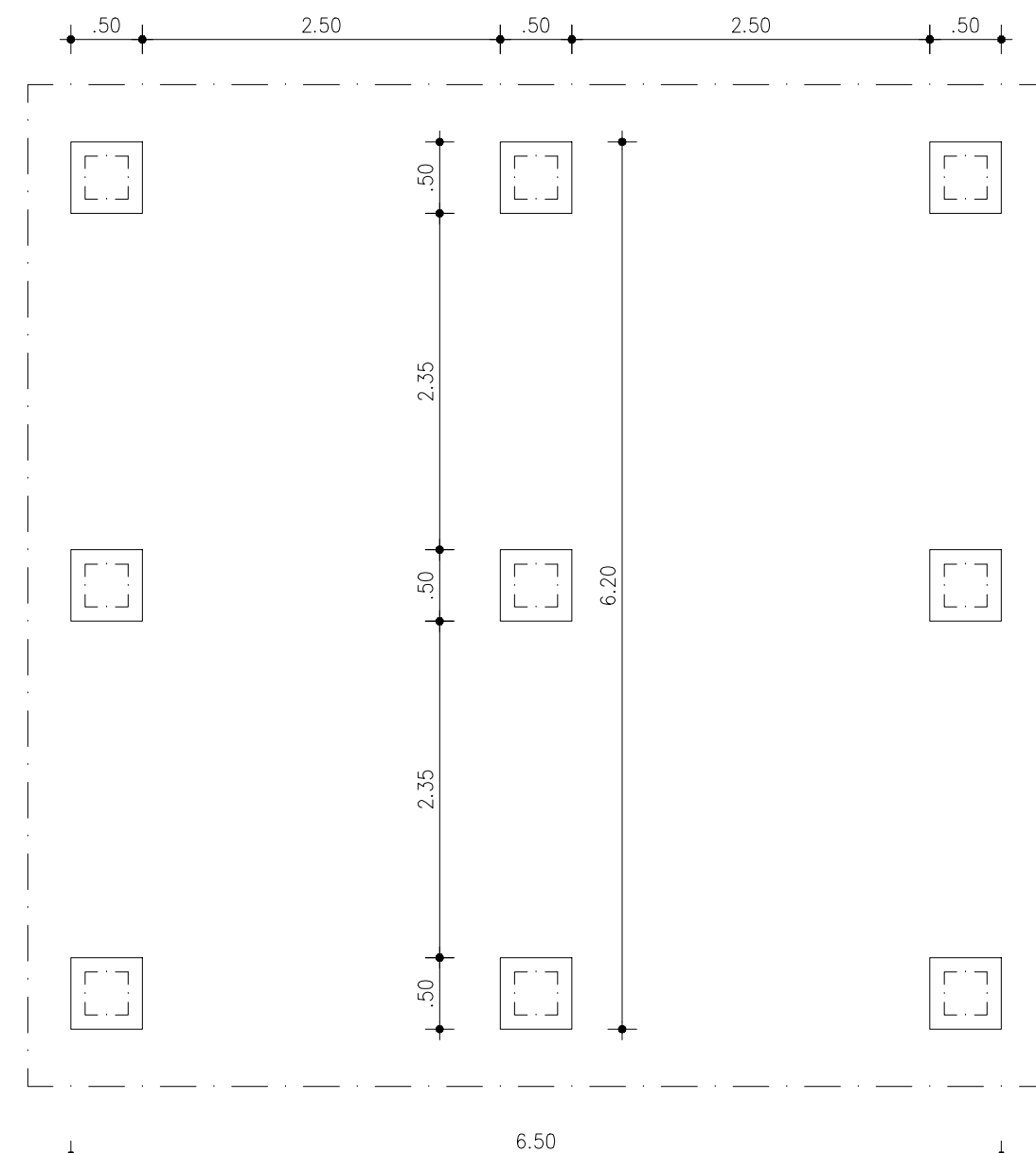
PERGOLADO JOGOS PLANTA BAIXA NIVEL FUNDAÇÃO
