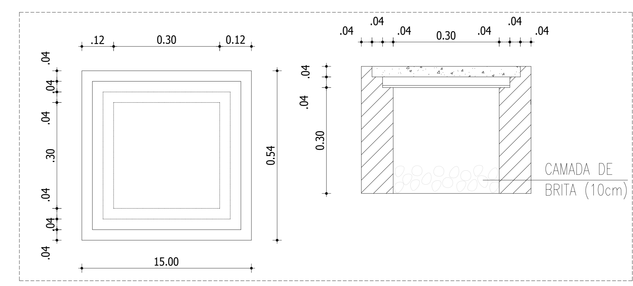
DETALHE CAIXA DE ALVENARIA 30X30X30 CM ESCALA S/E
