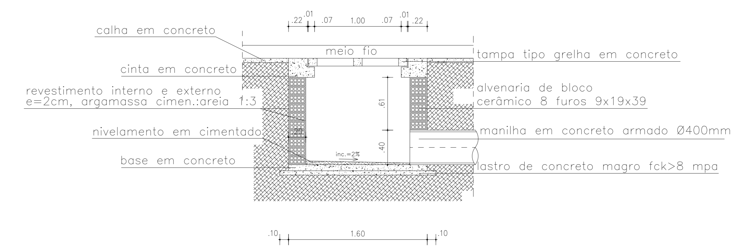
DETALHE BOCA DE LOBO SEÇÃO LONGITUDINAL ESCALA S/E
