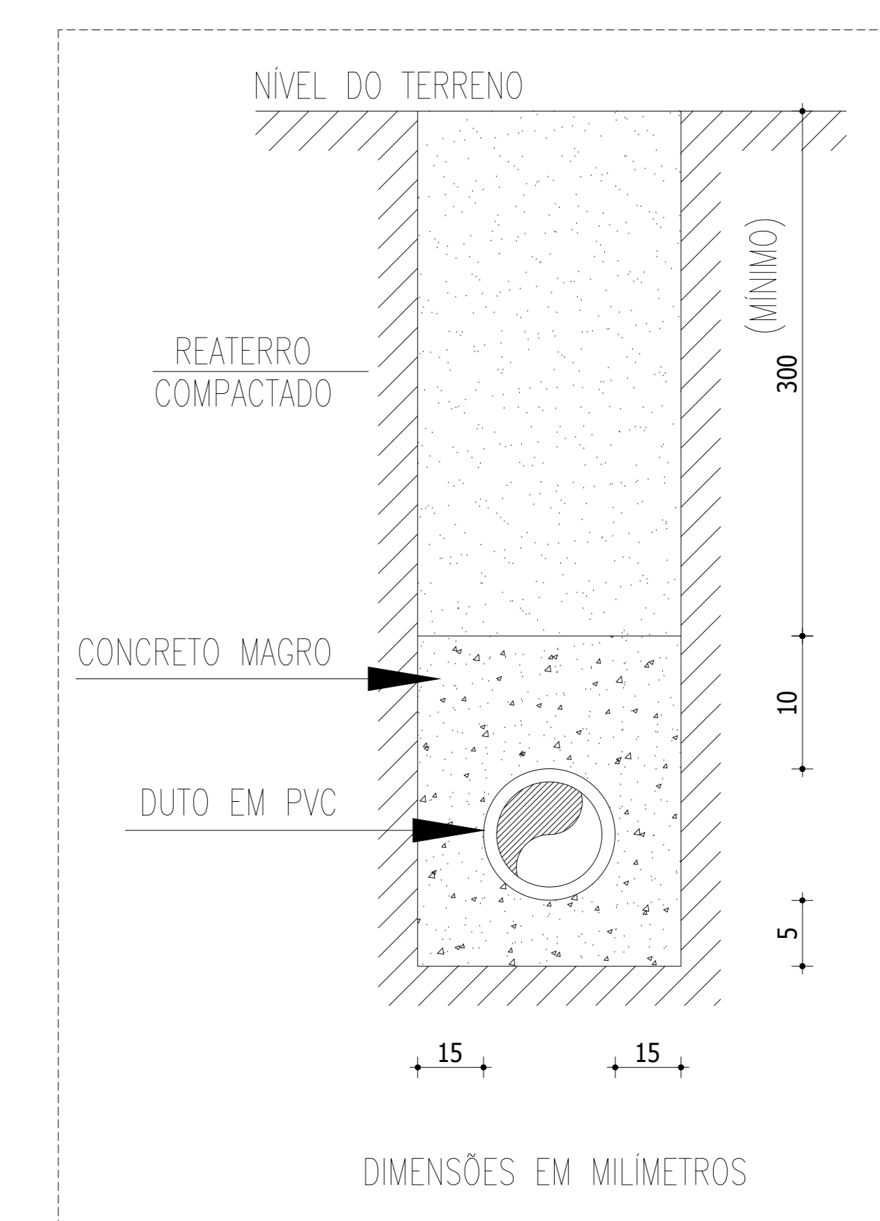
DETALHE ENVELOPAMENTO ESCALA S/E
