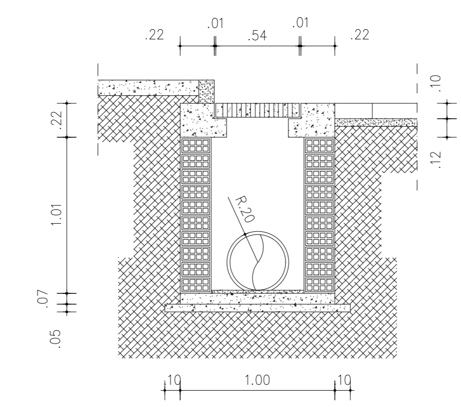
DETALHE BOCA DE LOBO SEÇÃO TRANSVERSAL ESCALA S/E
