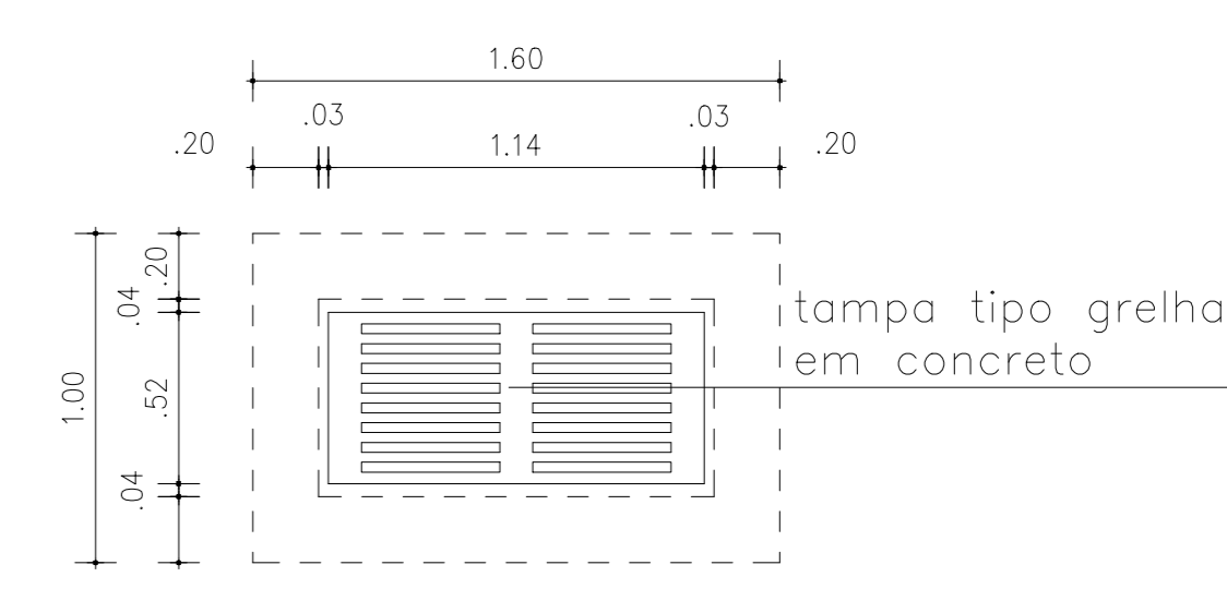
DETALHE BOCA DE LOBO PLANTA BAIXA ESCALA S/E
